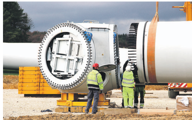
Im Inneren der Türme gibt es einen Aufzug (linkes Bild). Der Rotorstern – auf dem rechten Bild sieht man die Nabe – hat alleine einen Durchmesser von 117 Metern.
